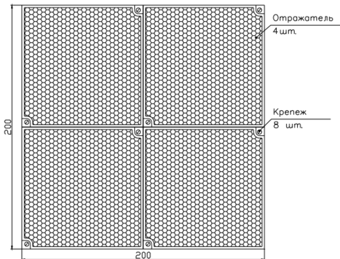
Рисунок А.2 - Монтаж четырех отражателей
